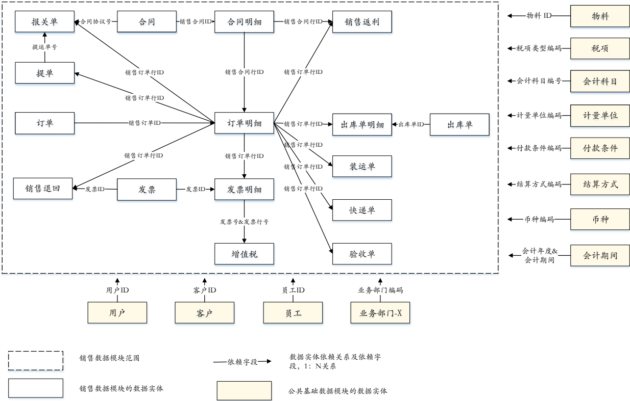
图1 销售数据实体关系图
